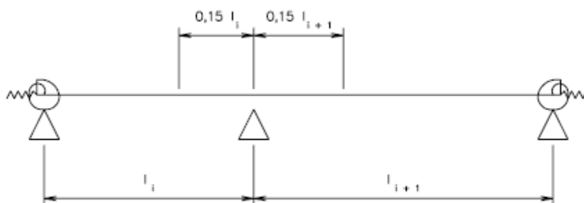
Figur 8.2 "Spennvidde" for kontinuerlige bruer
