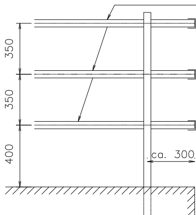
Figur 4.2 Rørrekkverk
