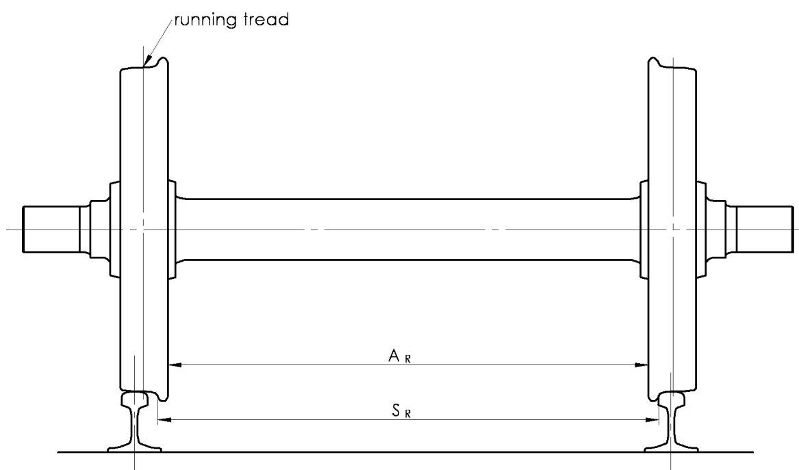
Figur 3b.1 Skisse som viser parametrene spesifisert i tabell 3.4.
