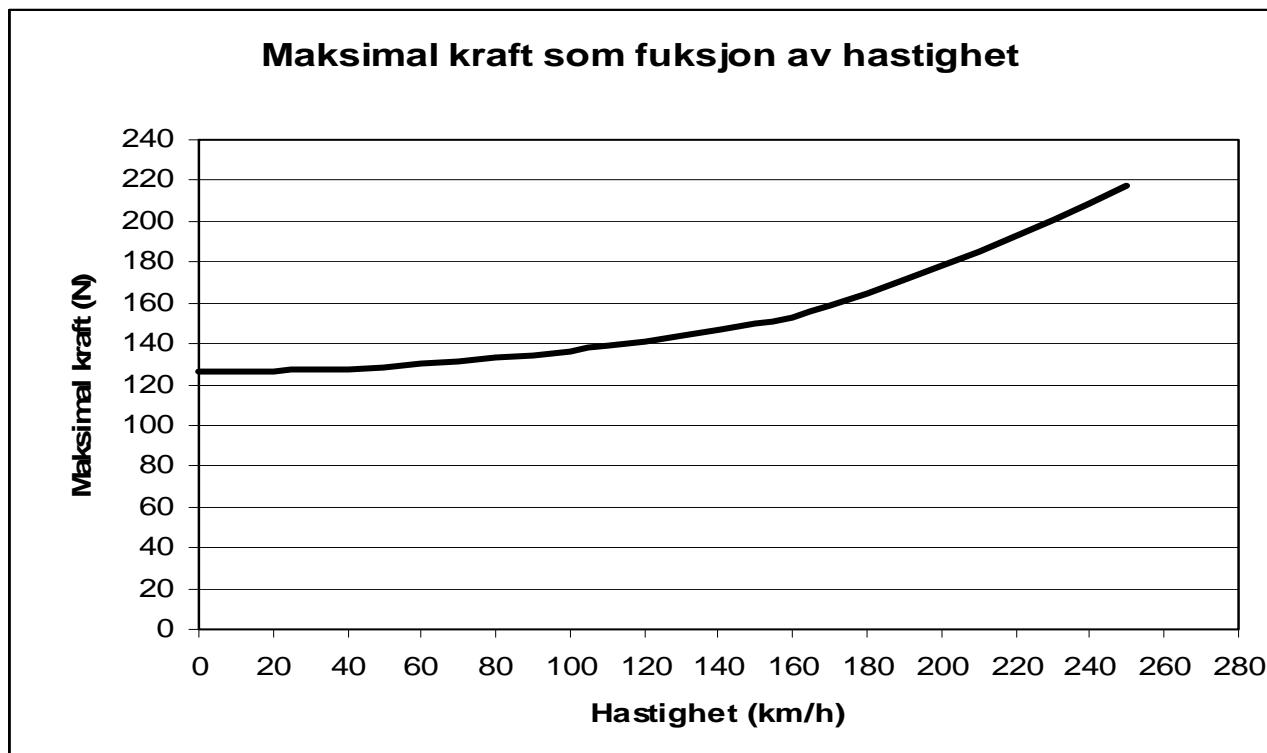
Figur 5.d.4 Grenseverdier for maksimal kraft som funksjon av hastighet.
