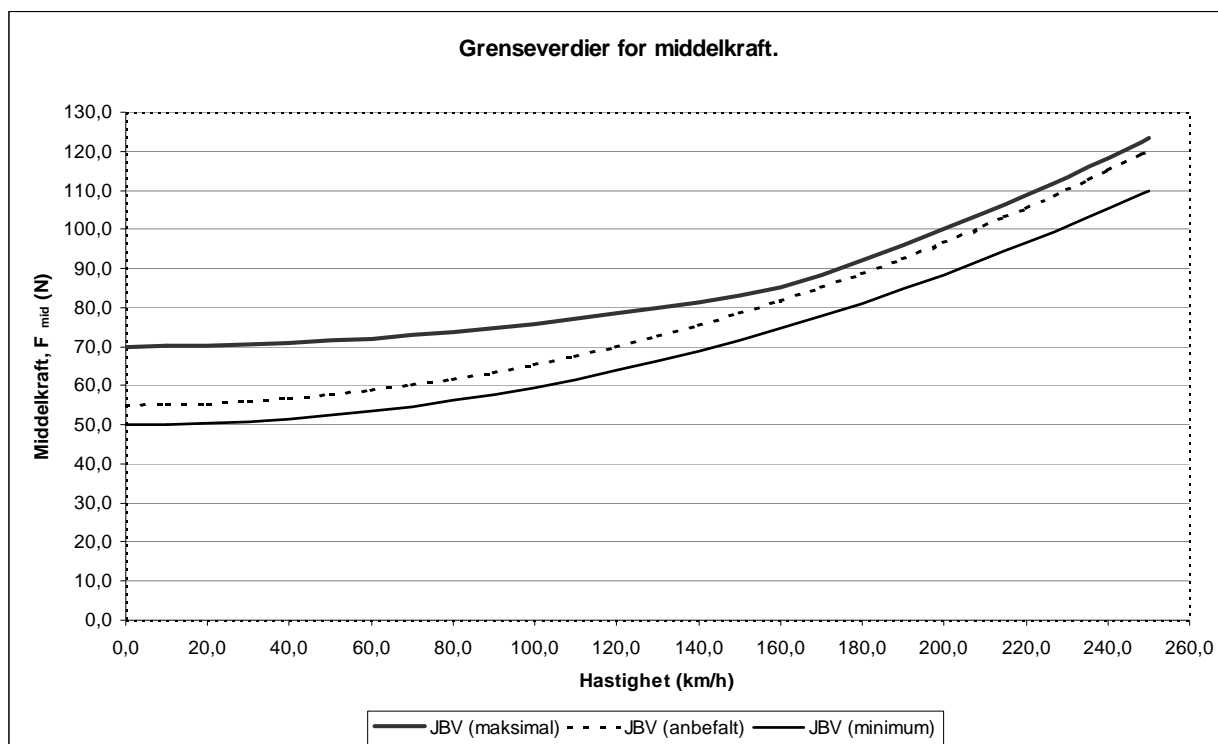
Figur 5.d.1 Middelkraft som funksjon av togfremføringshastighet.
