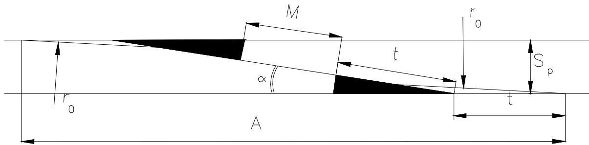
Figur 5.4 Sporsløyfe
