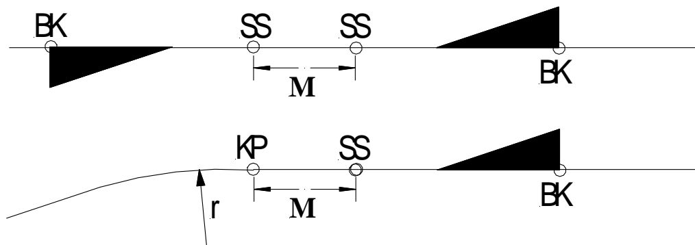
Figur 5.3 Krav til rettlinje M mellom to motstående veksler/veksel og curve
