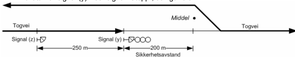
Figur 6.9 Samtidige togveier med sikkerhetsavstand 200 meter
