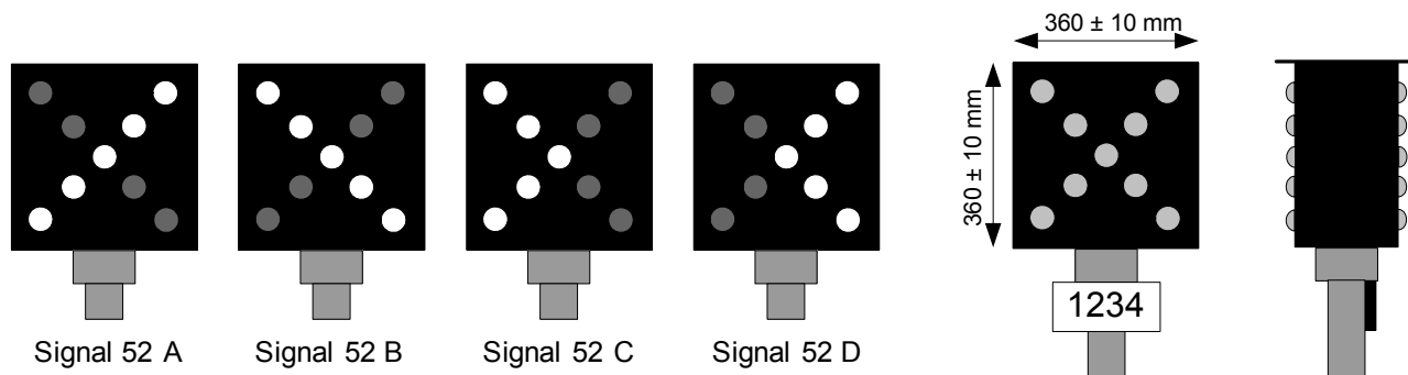
Figur 6.31 Sporvekselsignal for kryssvekselsignal - signalbilder og eksempel på lyssignal
