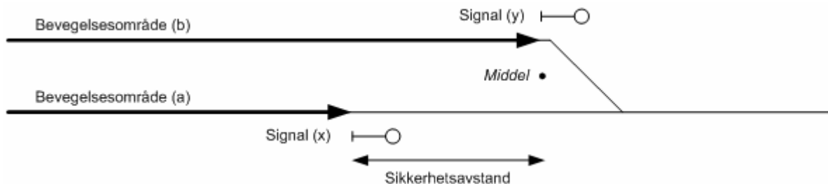
Figur 6.12 Parallele bevegelsesområder
