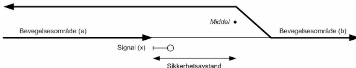
Figur 6.8 Bevegelsesområde mot flanken til en togvei
