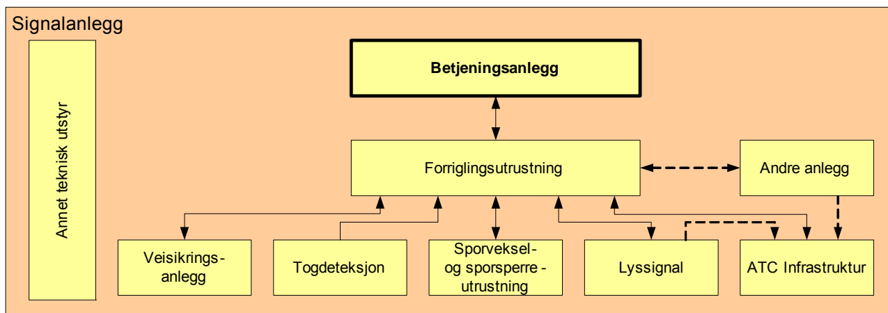
Figur 11.1 Systemoversikt signalanlegg
