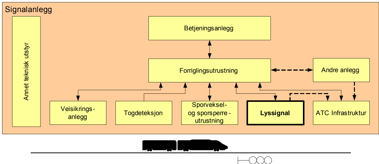
Figur 6.1 Systemoversikt signalanlegg
