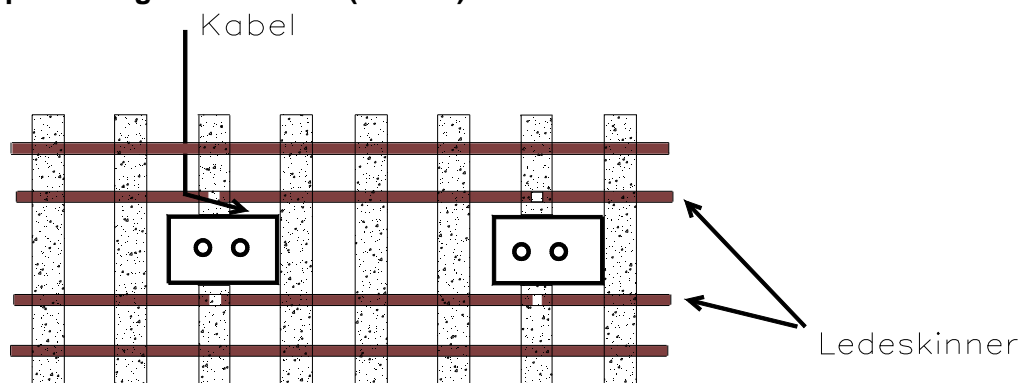
Figur 10.6 Plassering av balise i ledeskinner.
