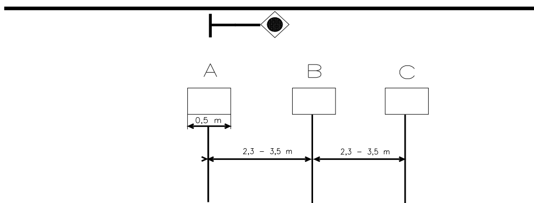
Figur 10.11 Eksempel på baliseplassering ved ATC forsignal.
