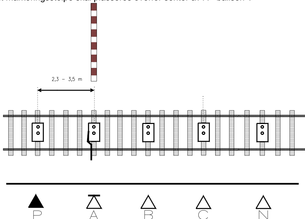
Figur 10.8 Plassering av markeringsstolpe ved balisegruppe.
