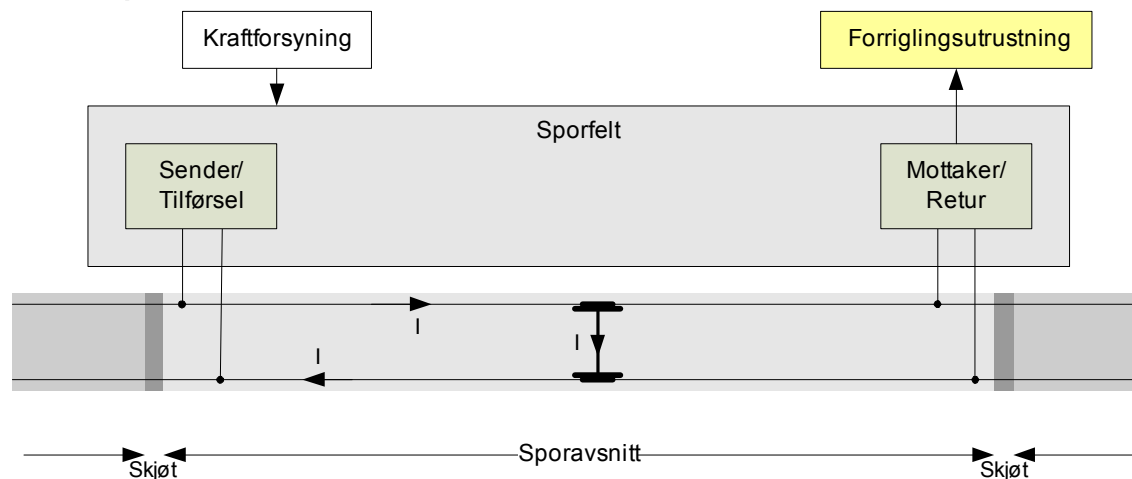
Figur 7.3 Systemdefinisjon - sporfelt
