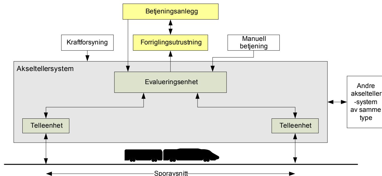
Figur 7.4 Systemdefinisjon - akseltellersystem
