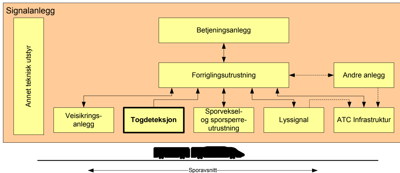
Figur 7.1 Systemoversikt signalanlegg
