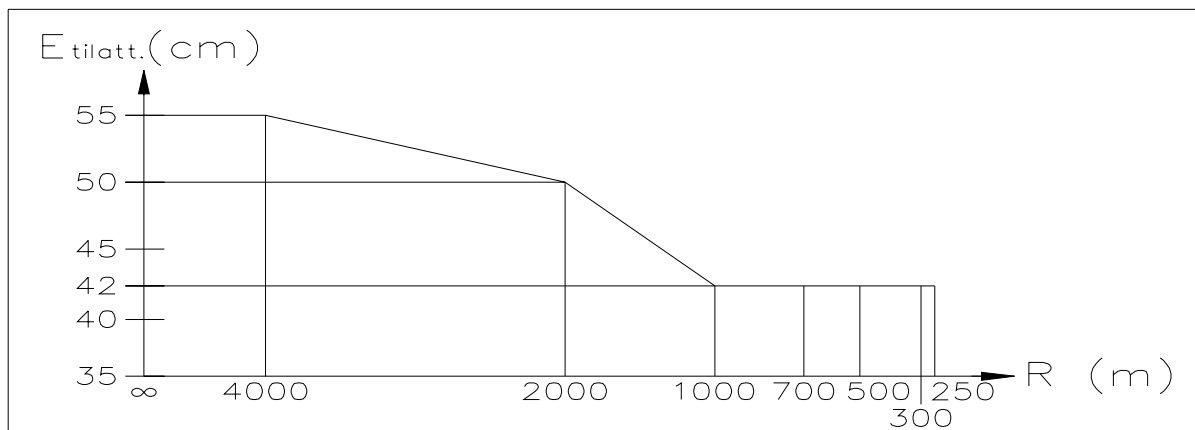
Figur 4 1 Vindutblåsningskurve for kontaktledningssystem med dimensjonerende hastighet opp til 200 km/h.
