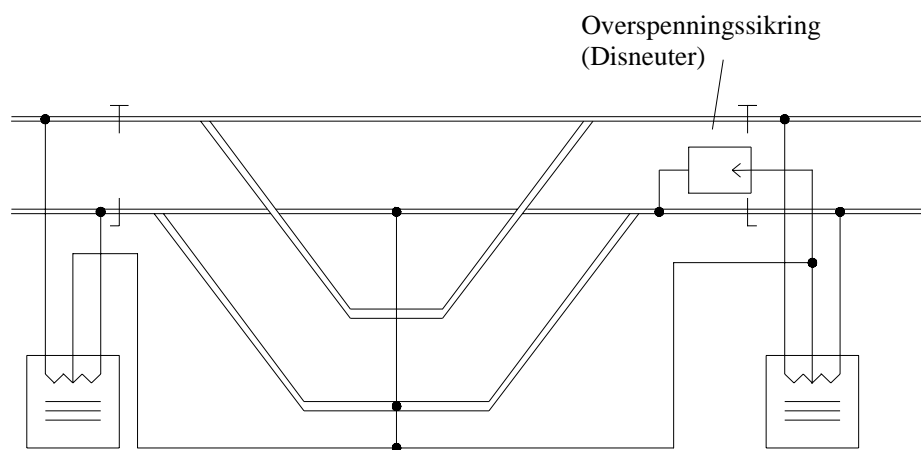
Figur 12.1 Returledning over stasjoner.
