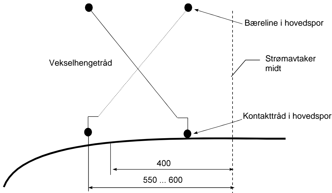
Figur 5.c.38 Vekselhengetrådets avstand fra spormid
