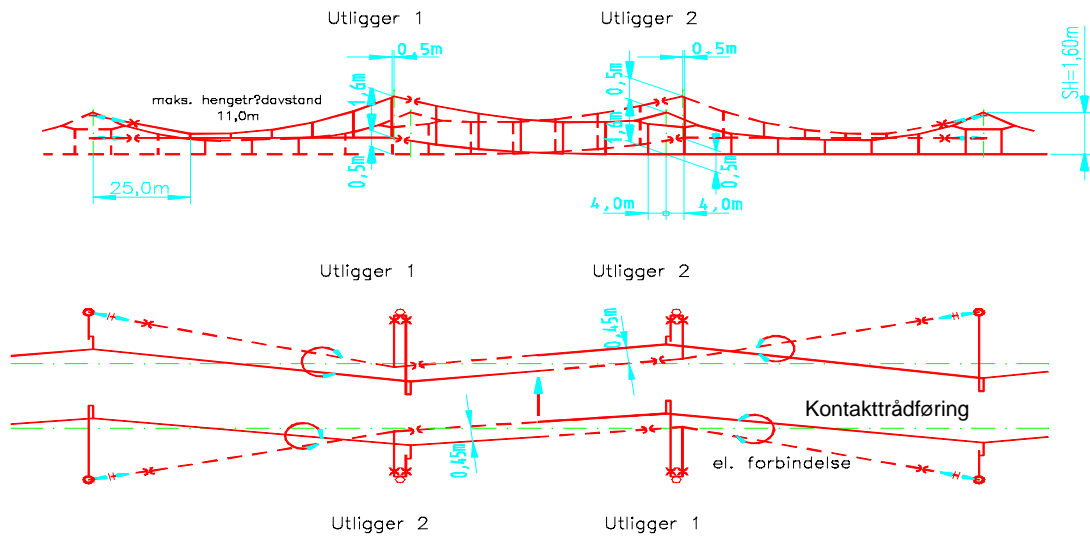
Figur 5.c.12 3-felts seksjon
