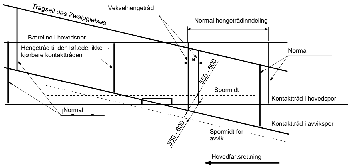
Figur 5.c.37 Plassering av vekselhengetråd i sporvekselområder
