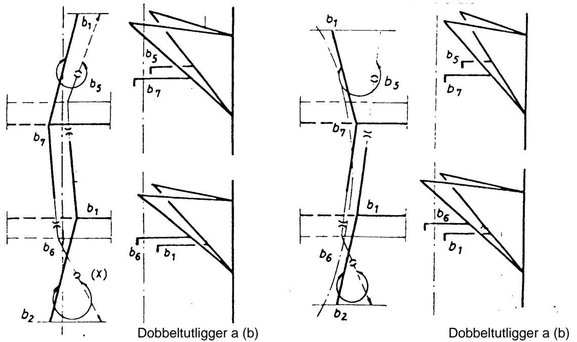
Figur 5.c.13 Anordning av utliggerne i seksjonsfelt
