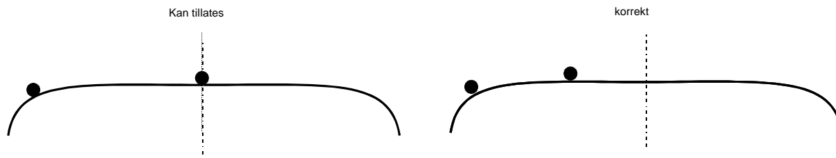
Figur 5.c.39 Krav til ledningsføring i vekslingsområdet
