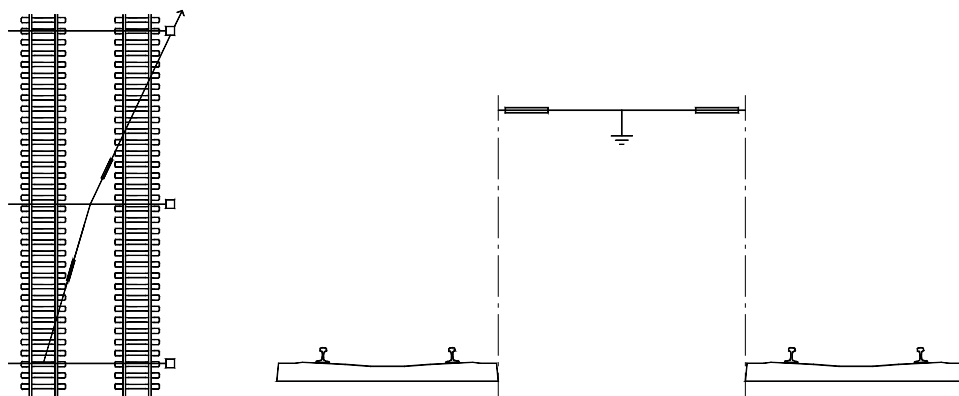
Figur 6.8. Elektrisk separasjon av kryssende ledninger
