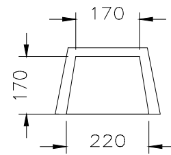
SNITT C-C
