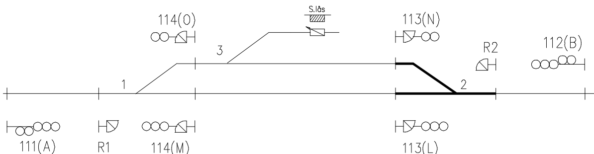
Figur 5.12 Forrigling av område for lokal skifting
