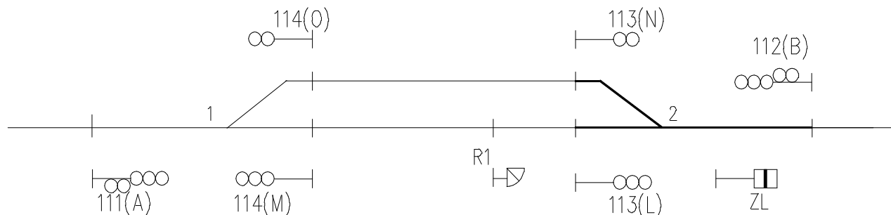
Figur 5.11 Forrigling av skifteområder.
